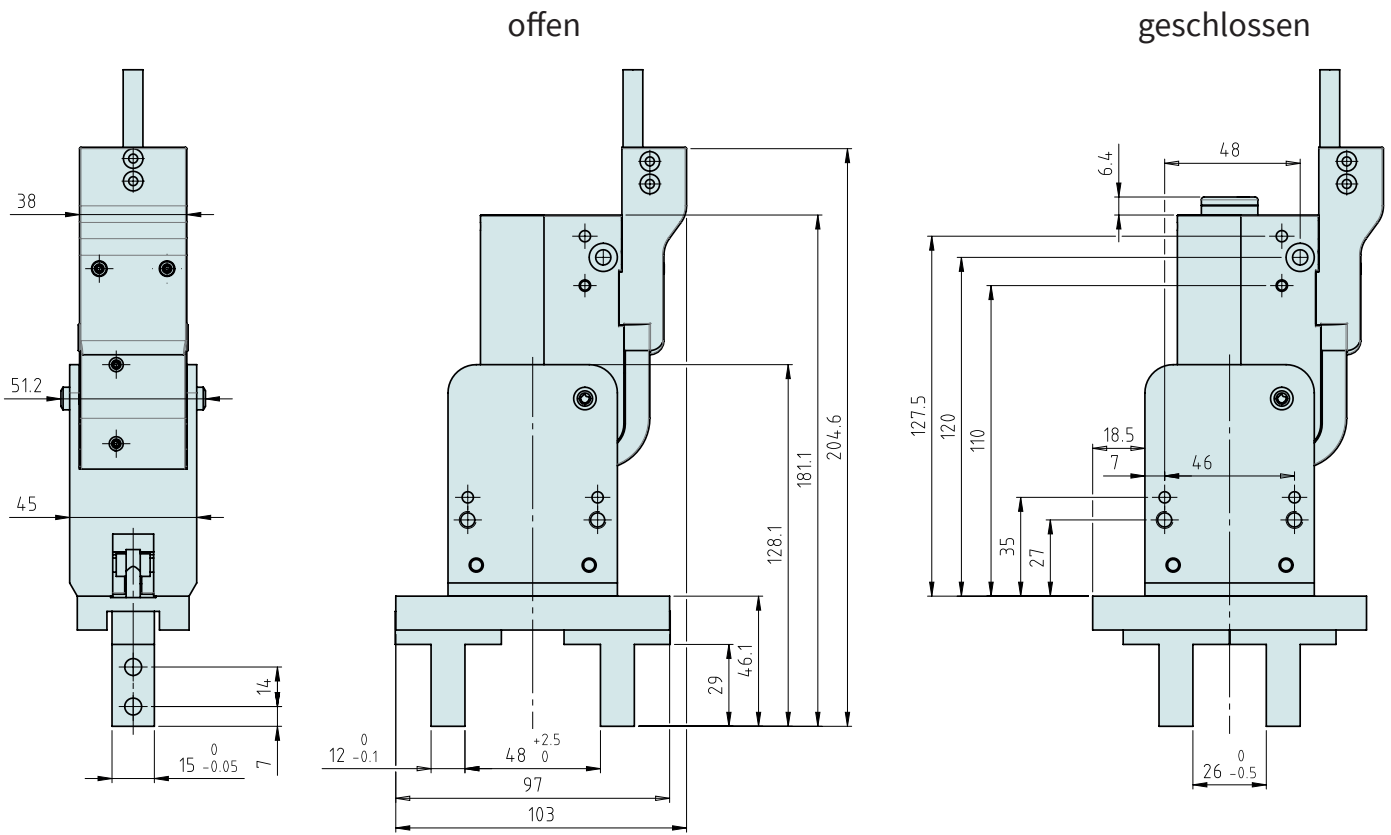
Abmessungen mm
